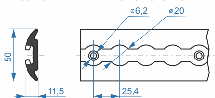
Listwa AIRLINE z zakończeniami
