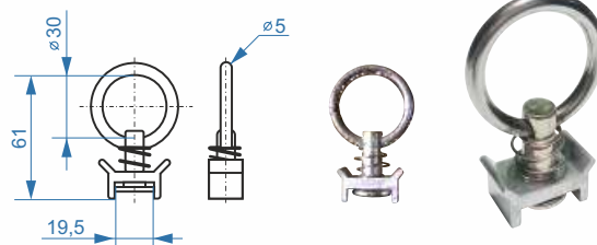
Uchwyt AIRLINE 400kg
