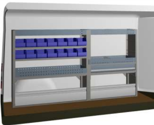
Zabudowa o wymiarach 1947 x 1100 x 382 mm Składa się z modułów: M2 + mM4
