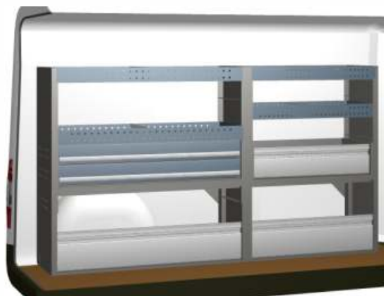
Zabudowa o wymiarach 1947 x 1100 x 382 mm Składa się z modułów: M6 + mM3
