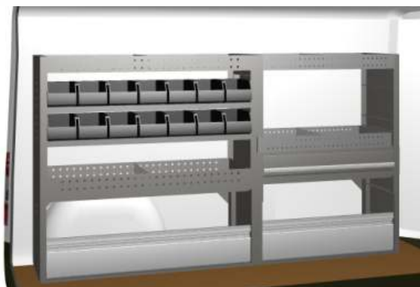
Zabudowa o wymiarach 1947 x 1100 x 382 mm Składa się z modułów: M2 + mM4
